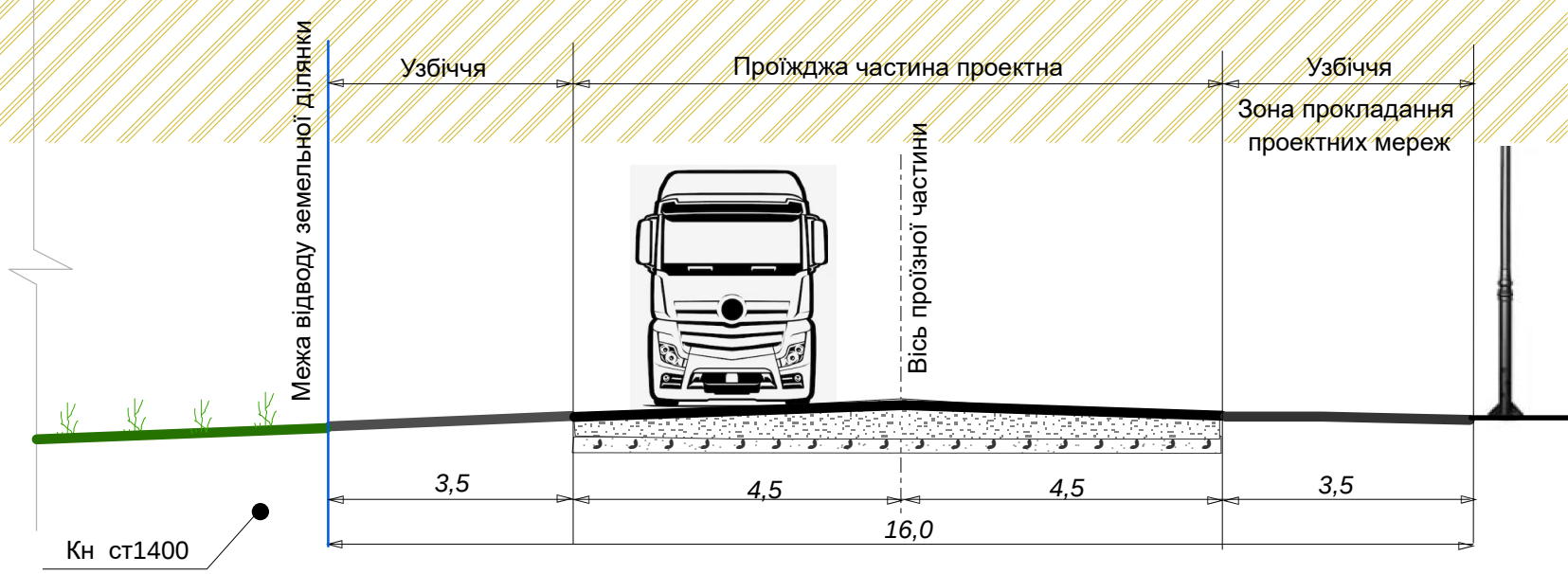
Поперечний профіль 1-1. М 1:100
